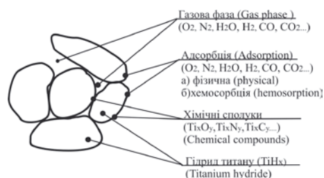
Рис.2 Схема розподілу домішок кисню, нітрогену, гідрогену та карбону в гідриді титану Fig. 2 The diagram of distribution of oxygen, nitrogen, hydrogen and carbon admixtures in titanium hydride
