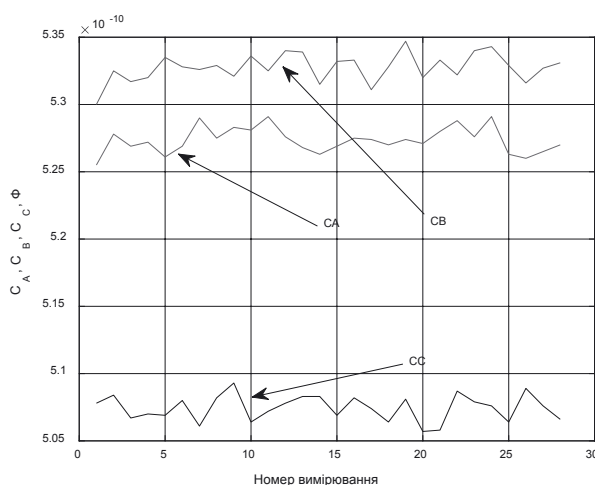
Рис. 2. Результати повторних вимірювань сукупних значень електричної ємності із застосуванням представленої на рис. 1а схеми обстеження
