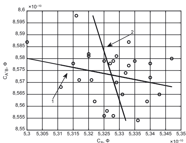
Рис. 6. Залежність між величинами електричної ємності, вимірюваними за застосування схеми обстеження ізоляції на рис. 1а та рис. 1б, та відповідні лінії регресії: 1 — лінія регресії C_B на C_{A-B} , 2 — лінія регресії C_{A-B} на C_B
