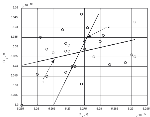
Рис. 5. Залежність між величинами електричної ємності, вимірюваними за застосування схеми обстеження ізоляції на рис. 1а, та відповідні лінії регресії: 1 — лінія регресії C_B на C_A , 2 — лінія регресії C_A на C_B
