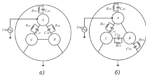
Рис. 1. Схеми обстеження ізоляції трьохжильних силових кабелів для формування системи рівнянь для оцінювання часткових ємностей із застосуванням сукупних вимірювань: а — за подавання випробувальної напруги на одну жилу силового кабелю; б — за подавання випробувальної напруги на дві жили силового кабелю
