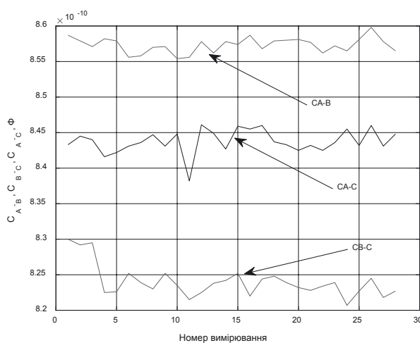
Рис. 3. Результати повторних вимірювань сукупних значень електричної ємності за застосування наведеної на рис. 1б схеми обстеження
